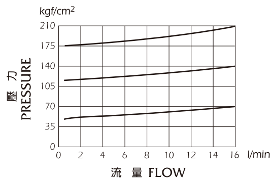
最低調整壓力特性 Min. Adj. PRESSURE
