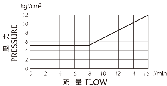
流量—壓力測試 NOMINAL OVERRIDE
